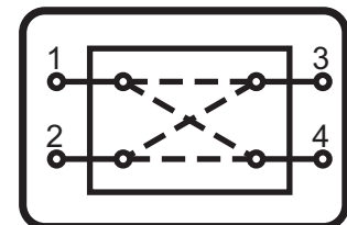
LLAVE DE CRUCE
