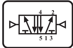
VÁLVULA BIESTABLE
