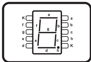
DISPLAY C.C.
