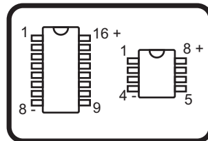
C.I.
