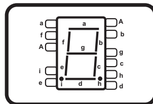
DISPLAY A.C.
