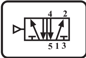
VÁLVULA MONOESTABLE
