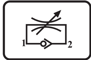
REGULADOR CAUDAL
