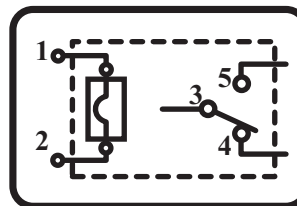
RELÉ
