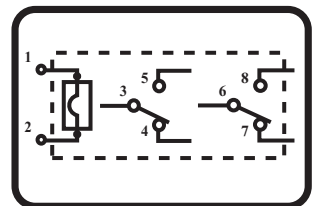
RELÉ 2 CTOS
