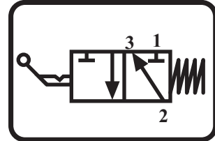
PALANCA
